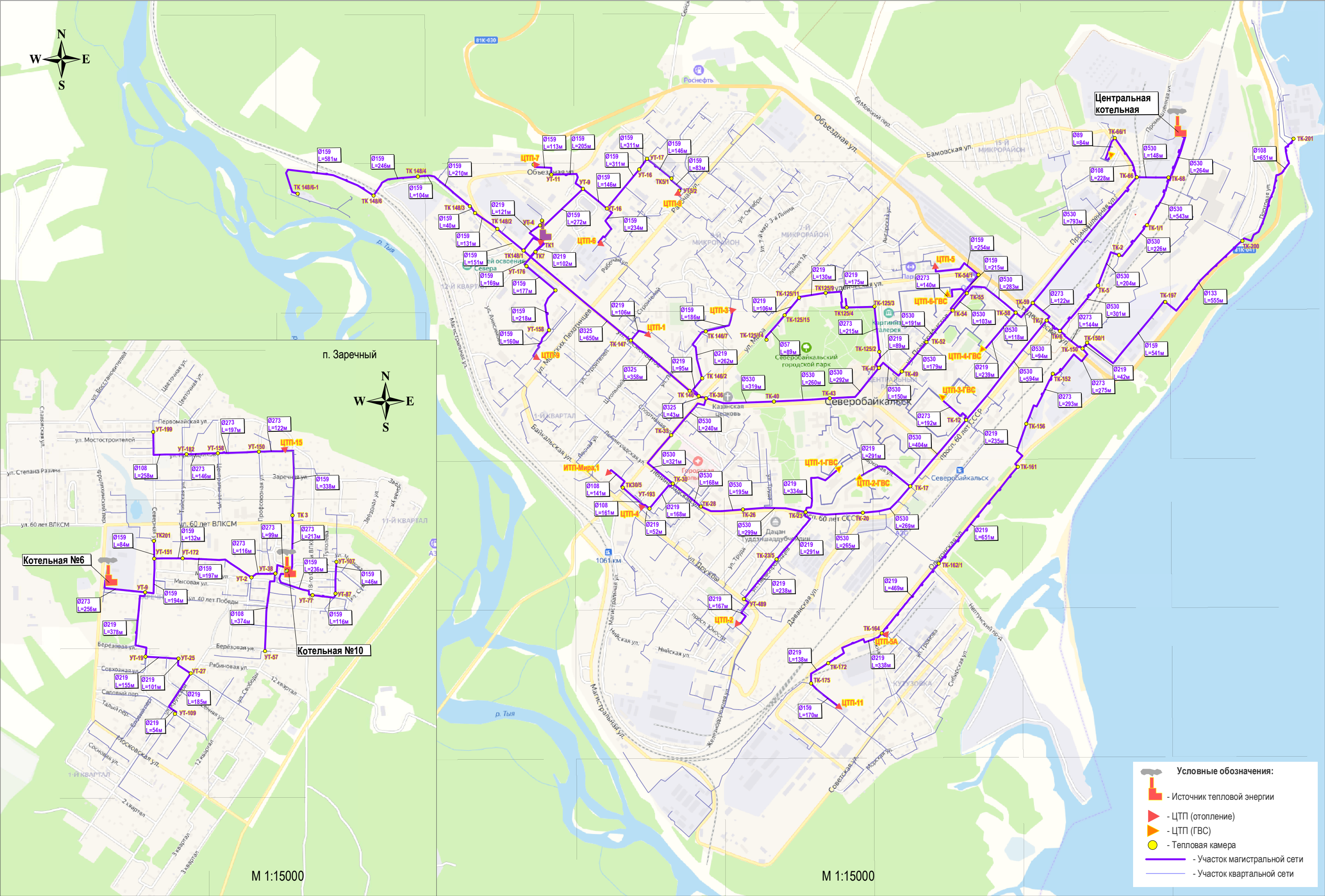
Приложение 5. Схема магистральных сетей от котельных МО "г.Северобайкальск"
