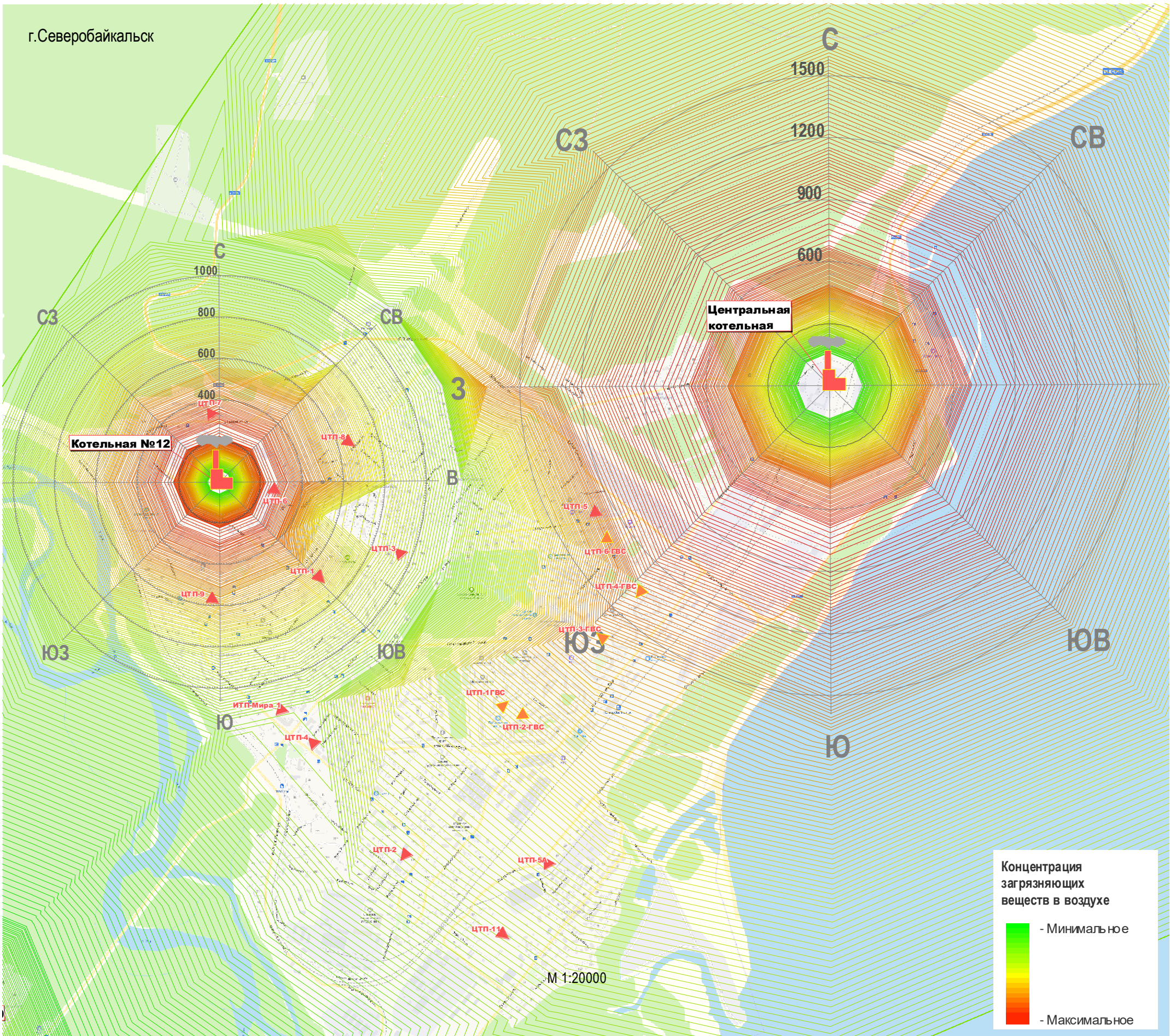
Приложение 5. Схема концентрации загрязняющих веществ в районе котельных МО "г.Северобайкальск"
