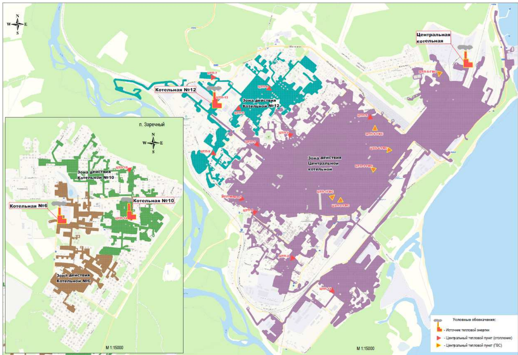
Рис. 2.1. Существующие зоны действия систем теплоснабжения и источников тепловой энергии в г. Северобайкальск и п. Заречный муниципального образования «город Северобайкальск».
