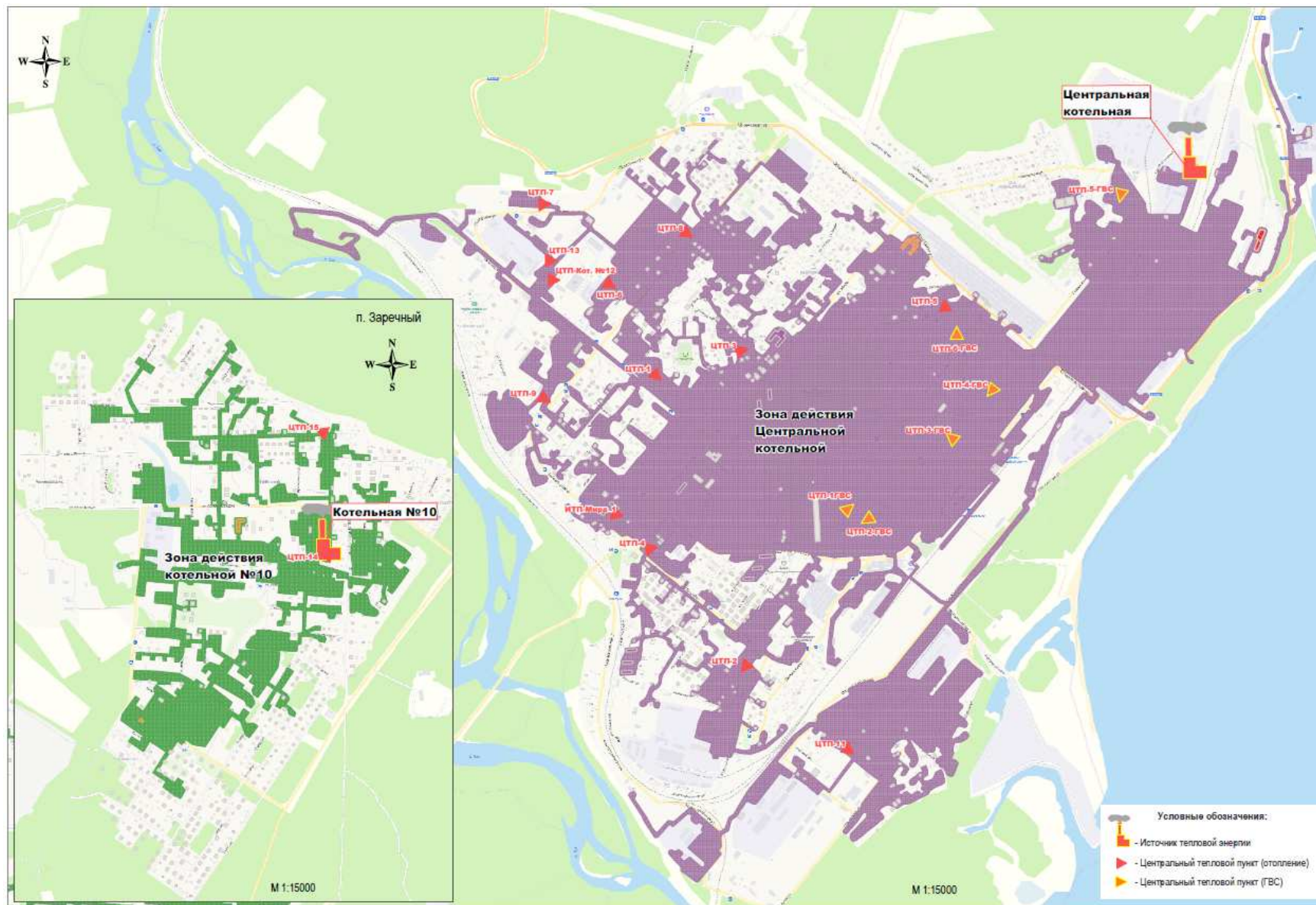
Рис. 2.2. Перспективные зоны действия систем теплоснабжения и источников тепловой энергии в г. Северобайкальск и п. Заречный муниципального образования «город Северобайкальск».
